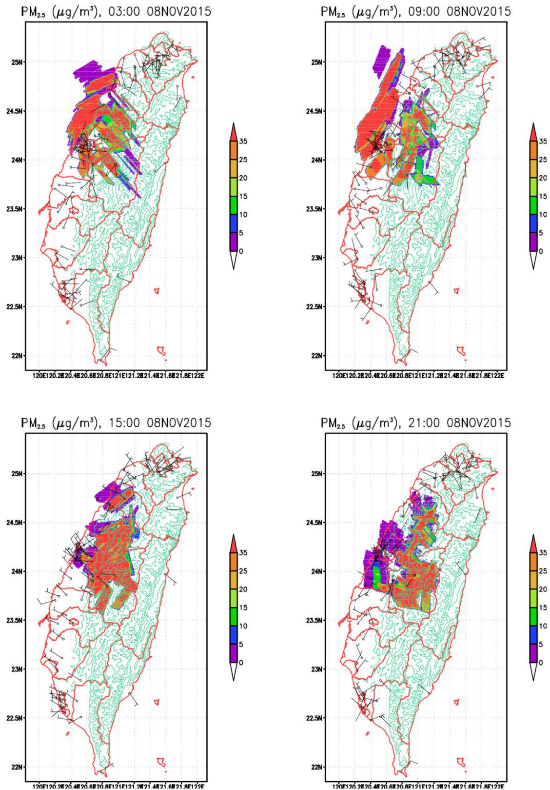
2015 年 11 月 08 日台中火力電廠、通霄火力電廠 3、9、15、21 時 之全台地區距地 20m 細懸浮粒濃度煙線圖 (事件日)
