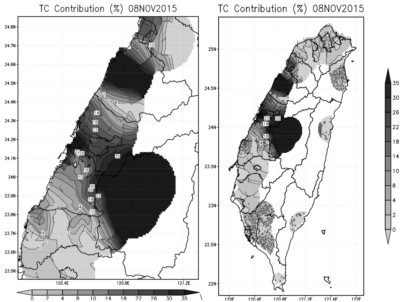
2015 年 11 月 08 日 台中火力電廠細懸浮微粒貢獻比例圖(事件日)
