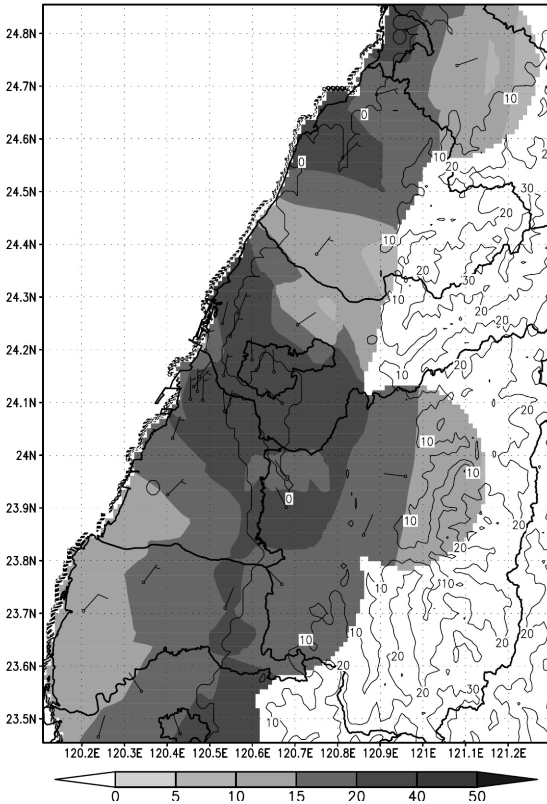
2015 年 11 月份風場及NO x (ppb) 月均值等濃度圖
