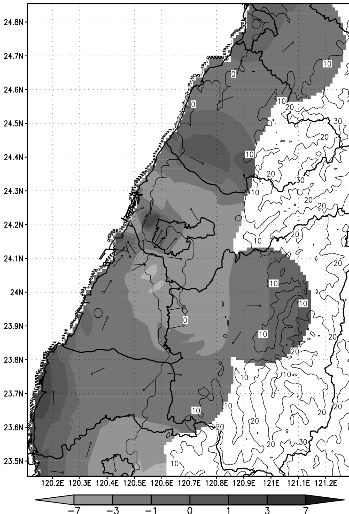
2015-(2010~2014)年 11 月NO x 月均值之濃度差值圖(單位：ppb)
