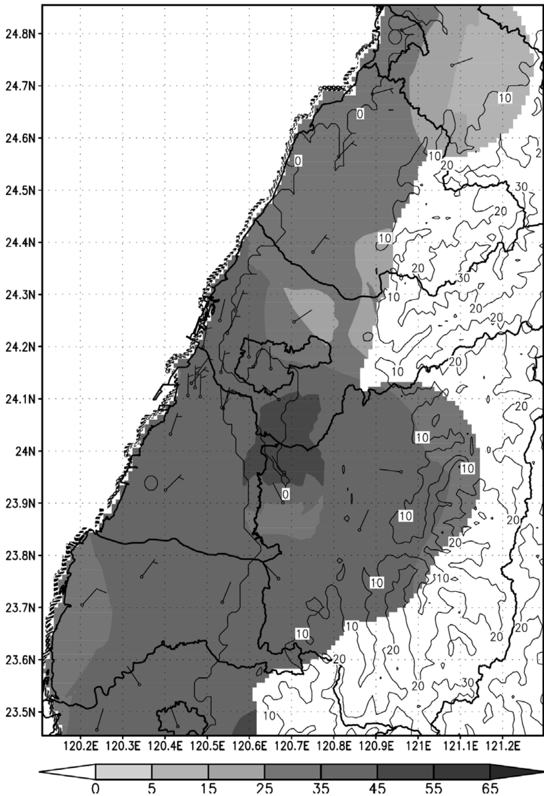
2015 年 11 月份風場及 PM_{2.5} ( \mu g/m^3 ) 月均值等濃度圖
