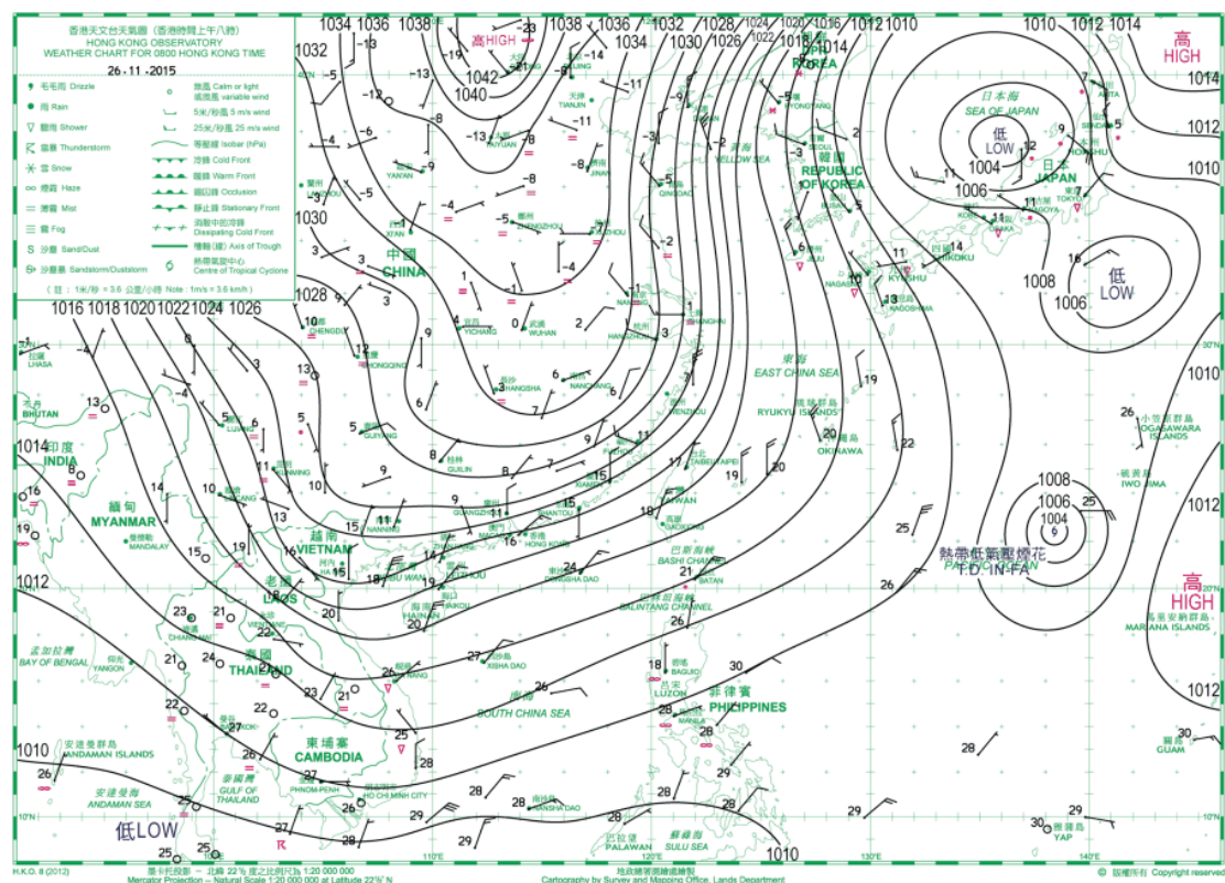
2015 年 11 月 26 日地面天氣圖(非事件日)
