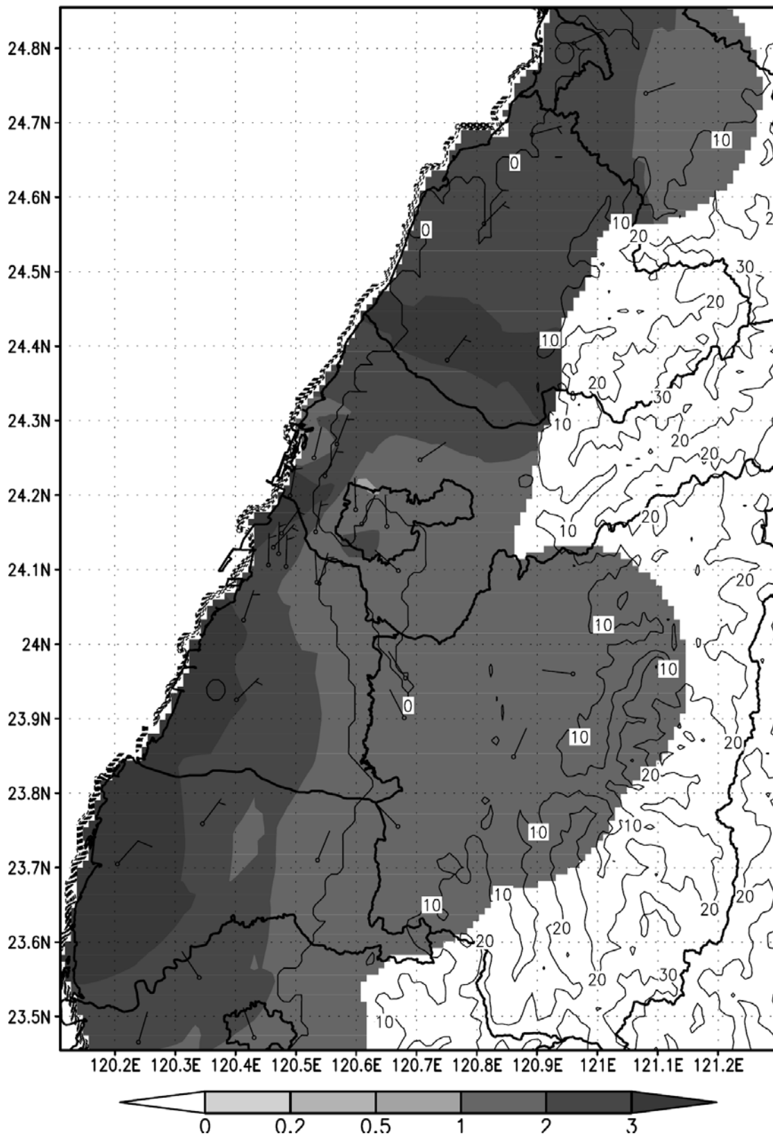
2015 年 11 月份風場及平均風速(m/s)等值圖
