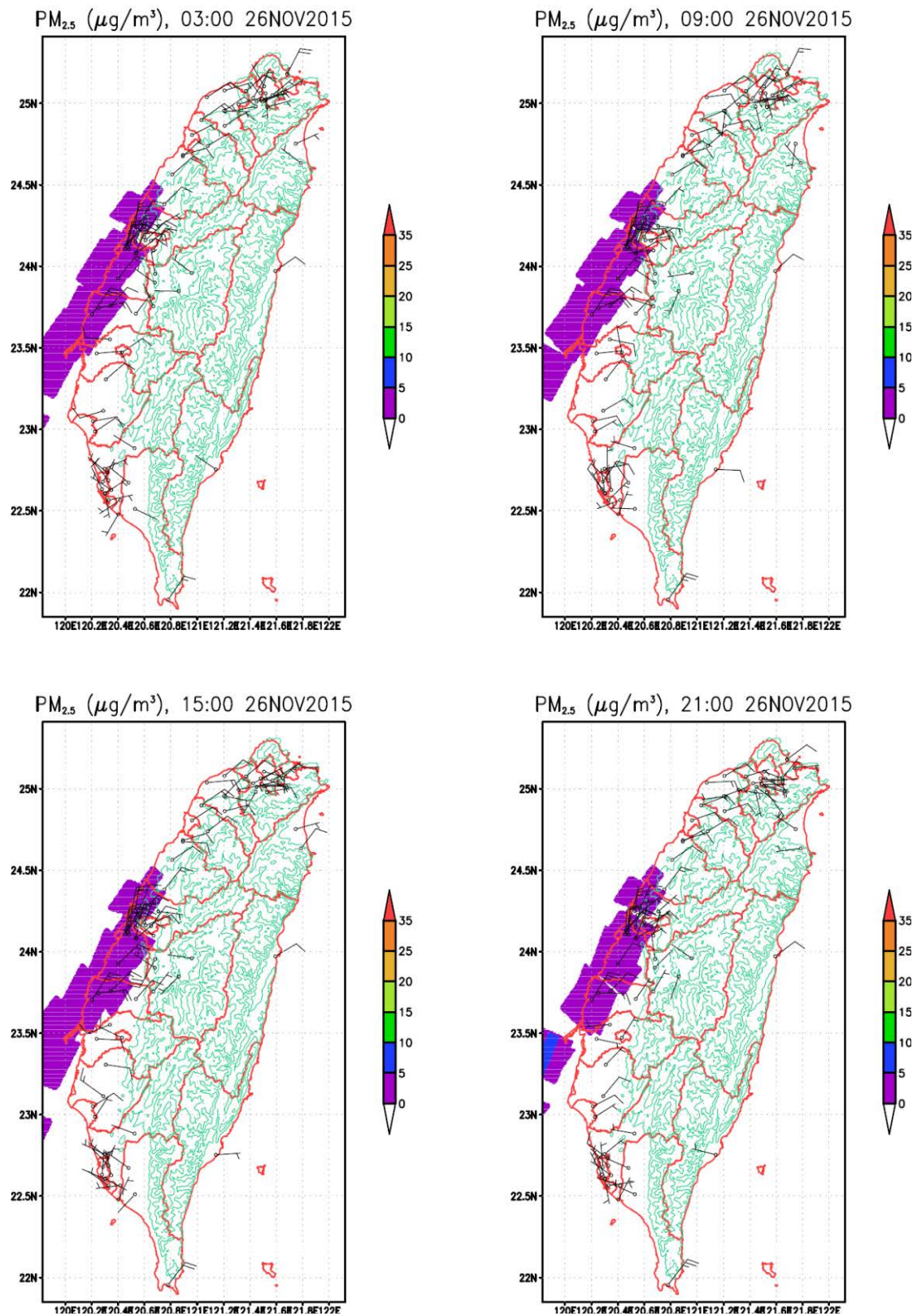
2015 年 11 月 26 日台中火力電廠、通霄火力電廠 3、9、15、21 時 之全台地區距地 20m 細懸浮粒濃度煙線圖 (非事件日)
