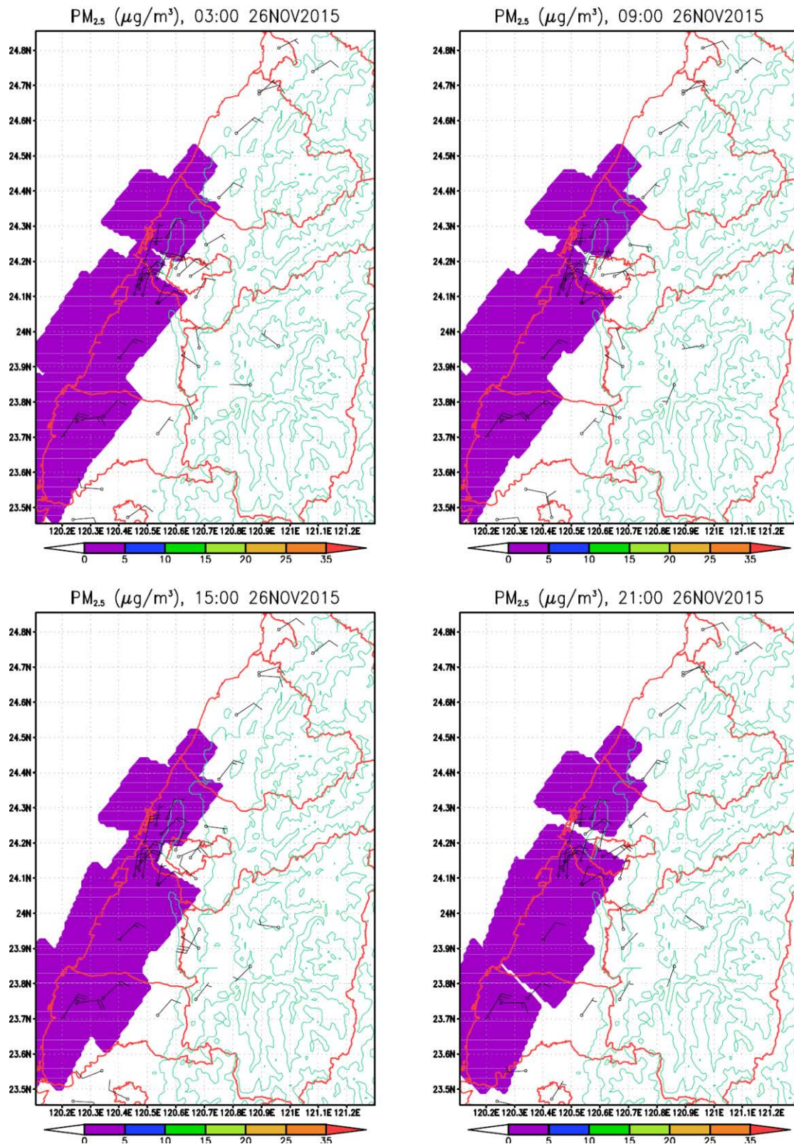
2015 年 11 月 26 日台中火力電廠、通霄火力電廠 3、9、15、21 時 之中部地區距地 20m 細懸浮粒濃度煙線圖 (非事件日)
