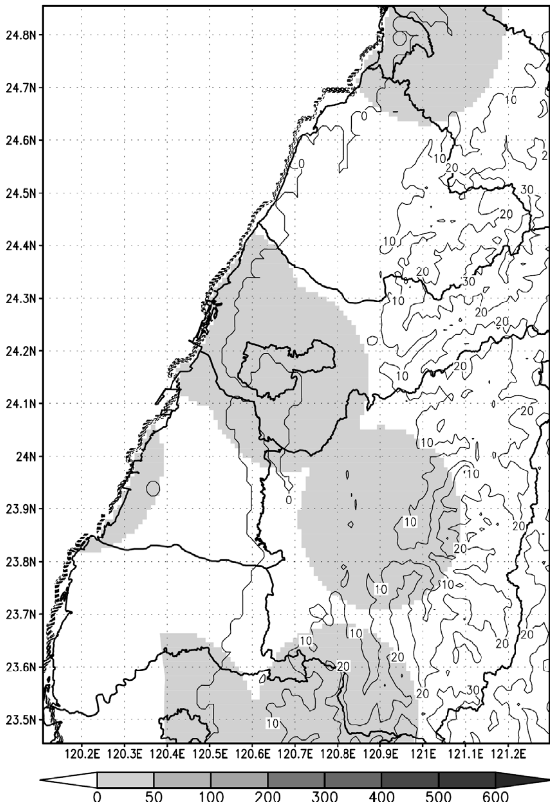
2015 年 11 月份風場及累積雨量(mm)圖
