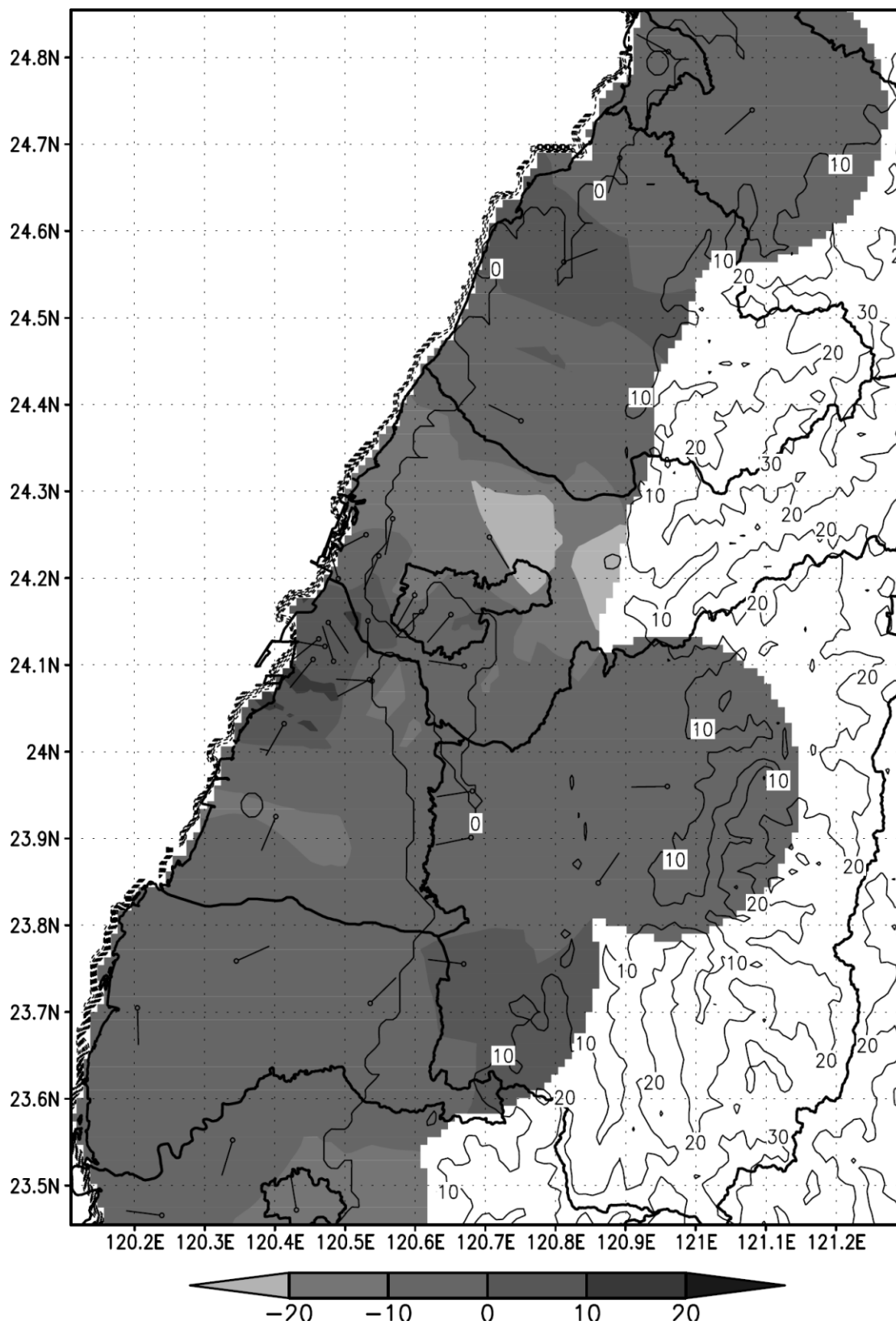
2015-(2010~2014)年 11 月 PM 10 月均值之濃度差值圖(單位： \mu\text{g}/\text{m}^3 )
