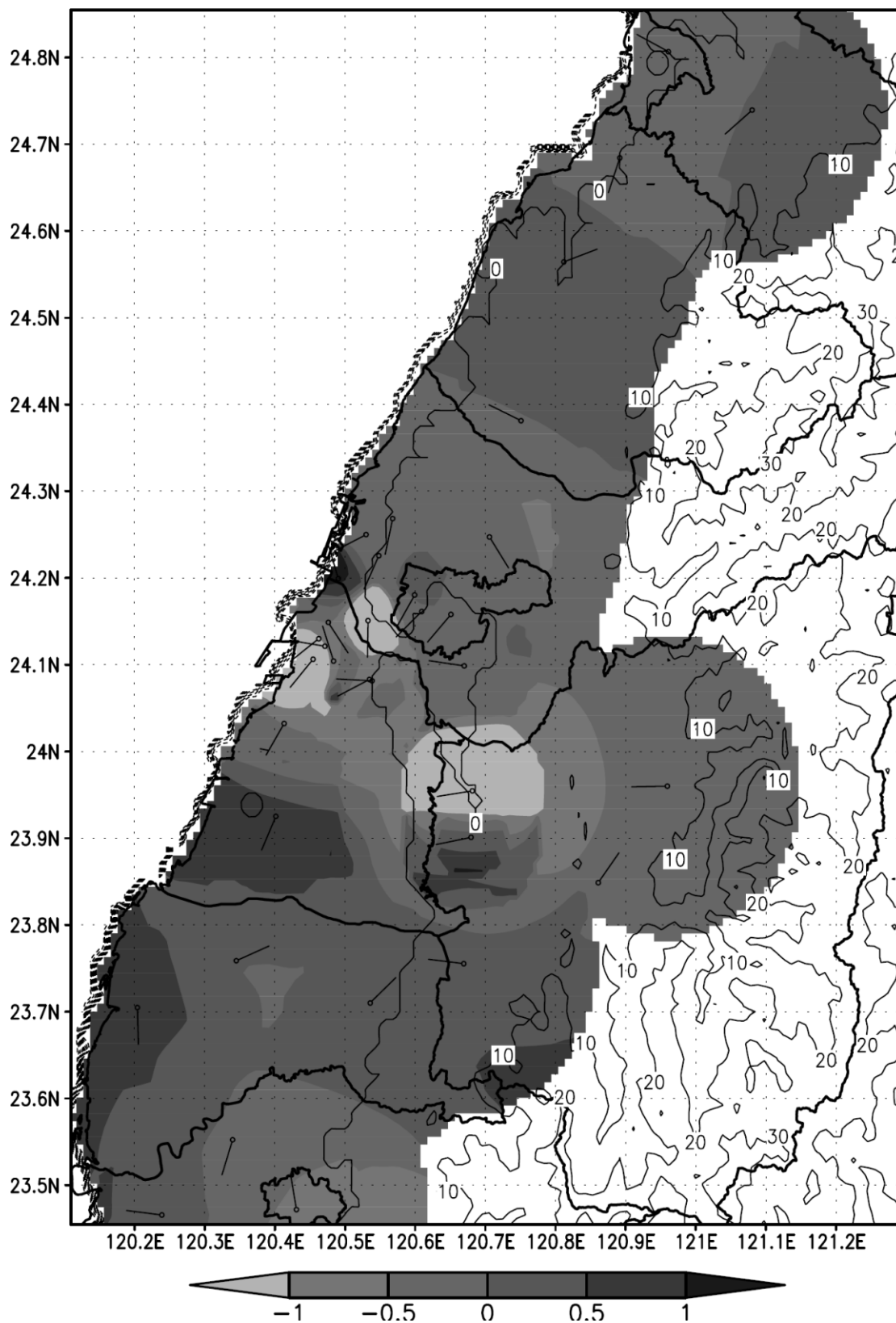
2015-(2010~2014)年 11 月SO 2 月均值之濃度差值圖(單位：ppb)
