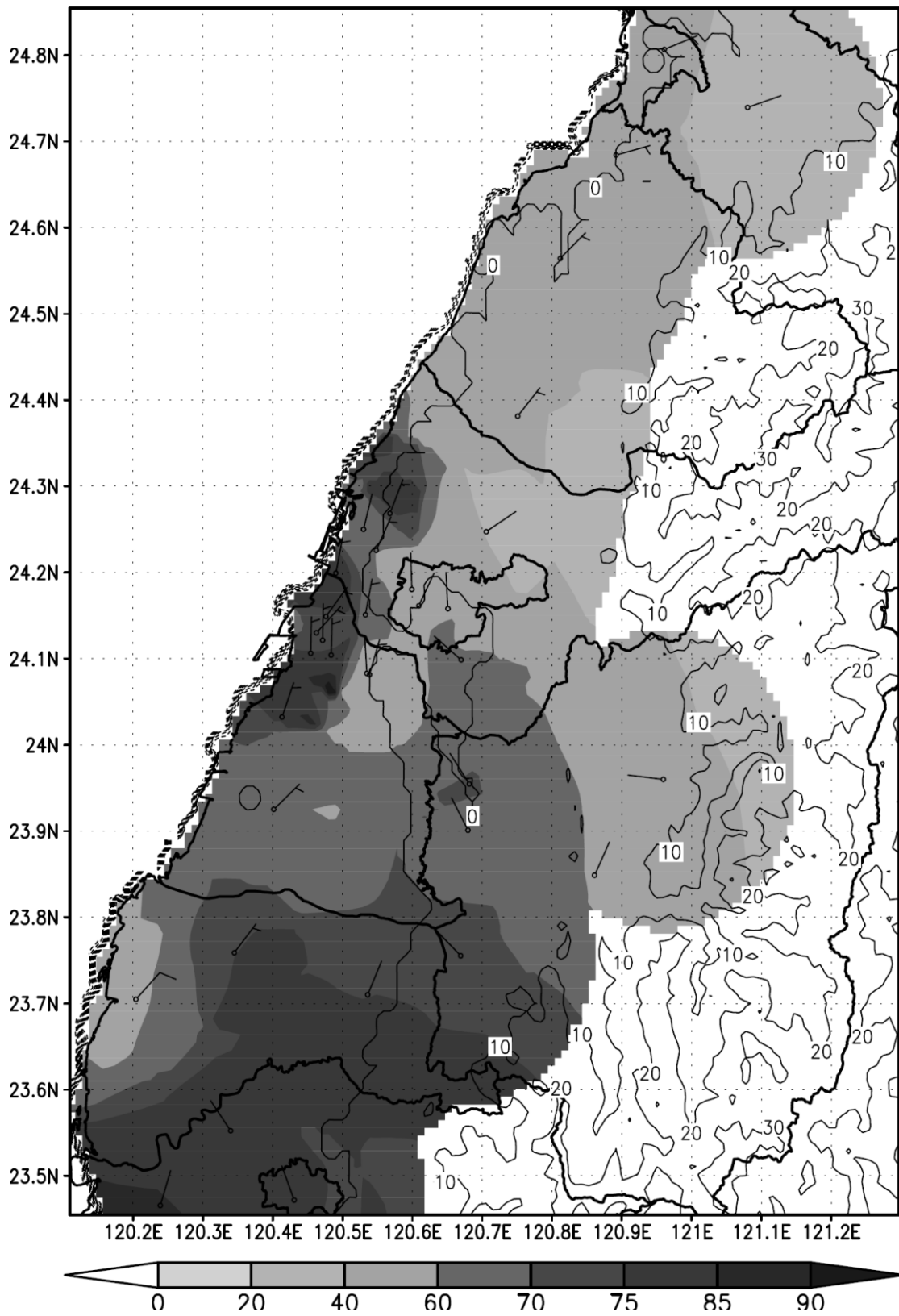
2015 年 11 月份風場及 PM_{10} ( \mu g/m^3 ) 月均值等濃度圖
