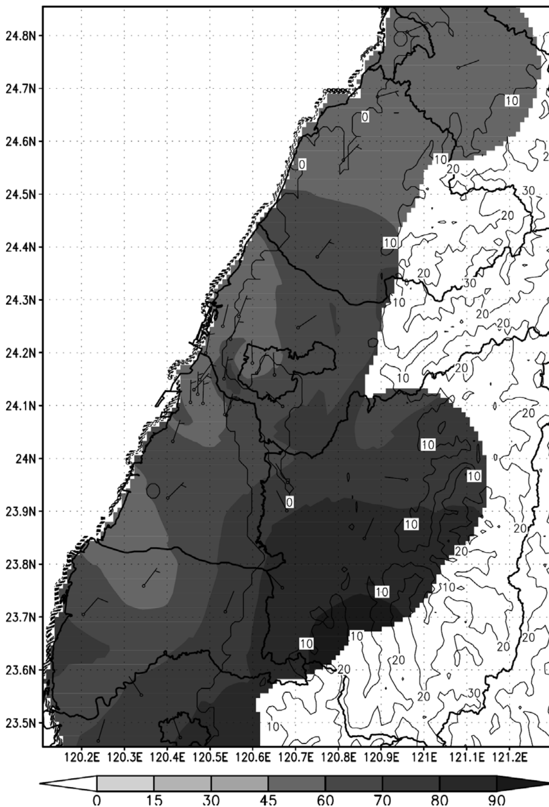
2015 年 11 月份風場及O 3 (ppb)小時最大值等濃度圖
