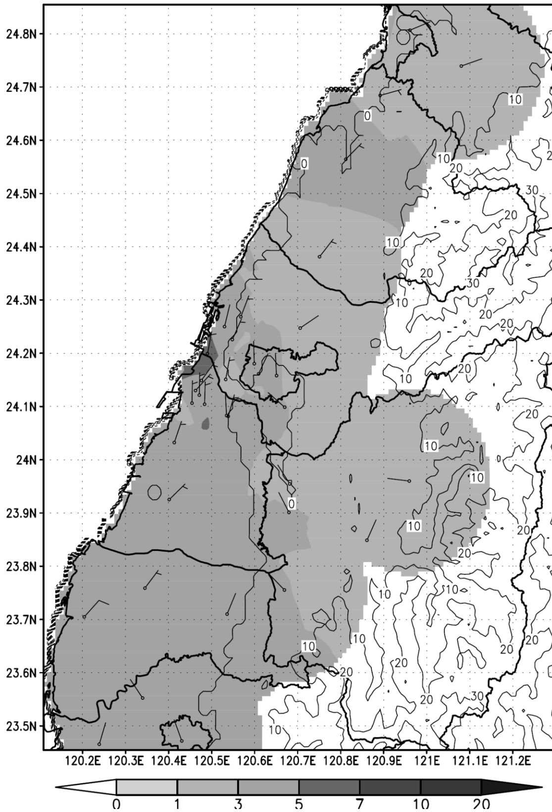
2015 年 11 月份風場及SO 2 (ppb) 月均值等濃度圖
