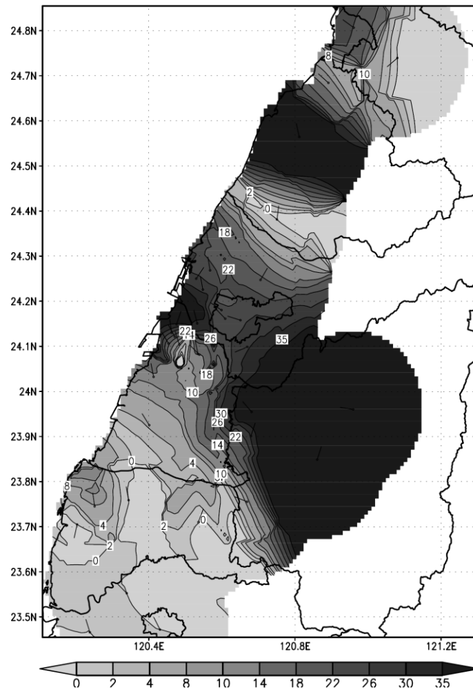
2015 年 11 月 08 日台中電廠+通霄電廠細懸浮微粒貢獻比例圖(事件日)
