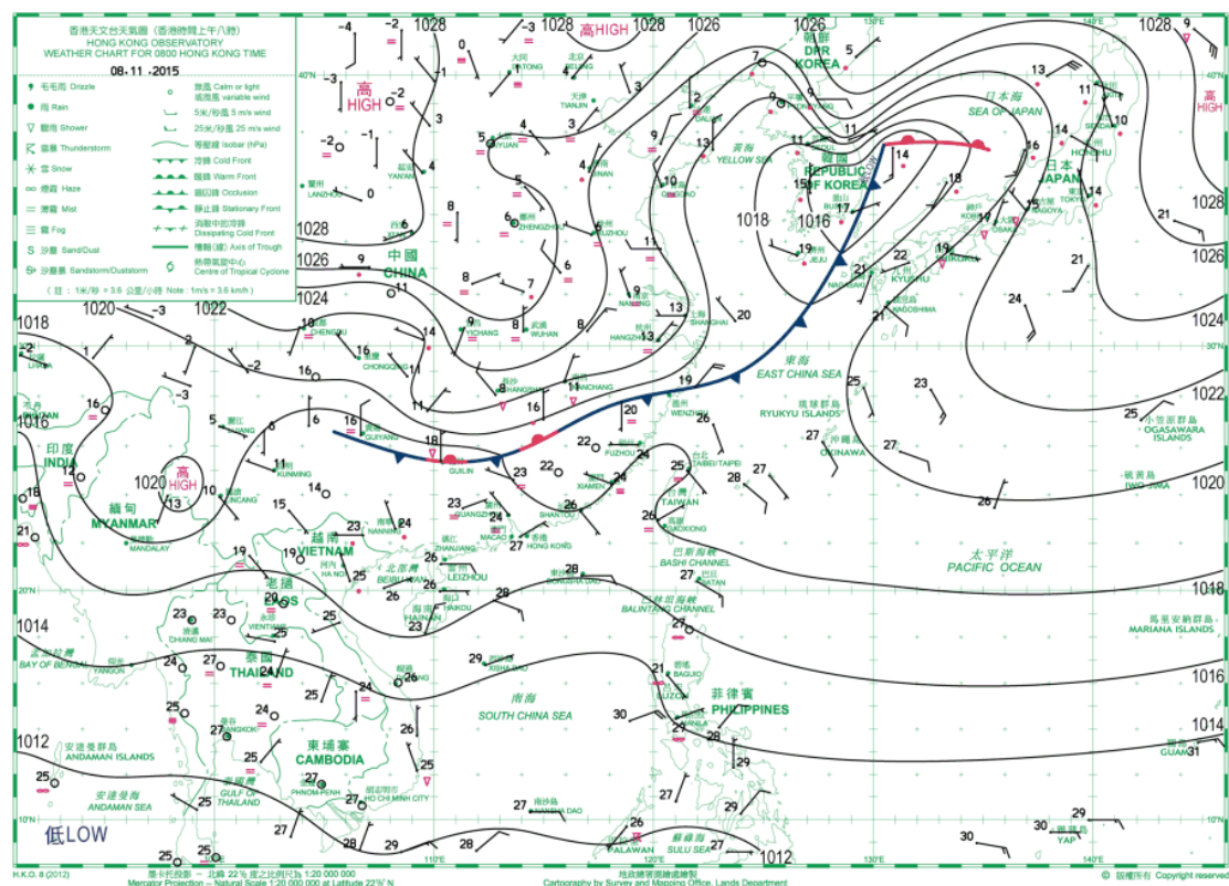
2015 年 11 月 08 日地面天氣圖(事件日)
