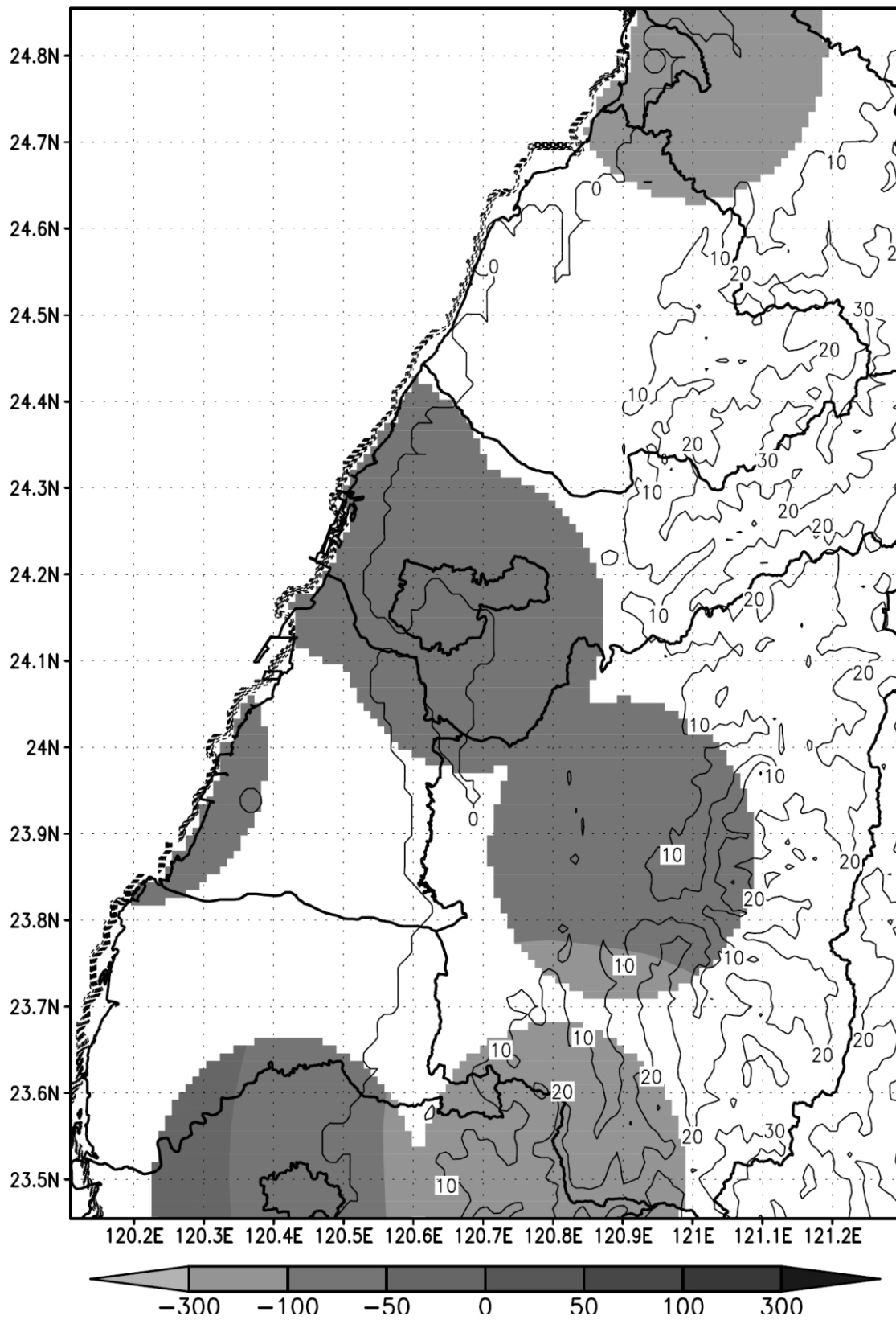
2015-(2010~2014)年 11 月累積雨量差值圖(單位：mm)
