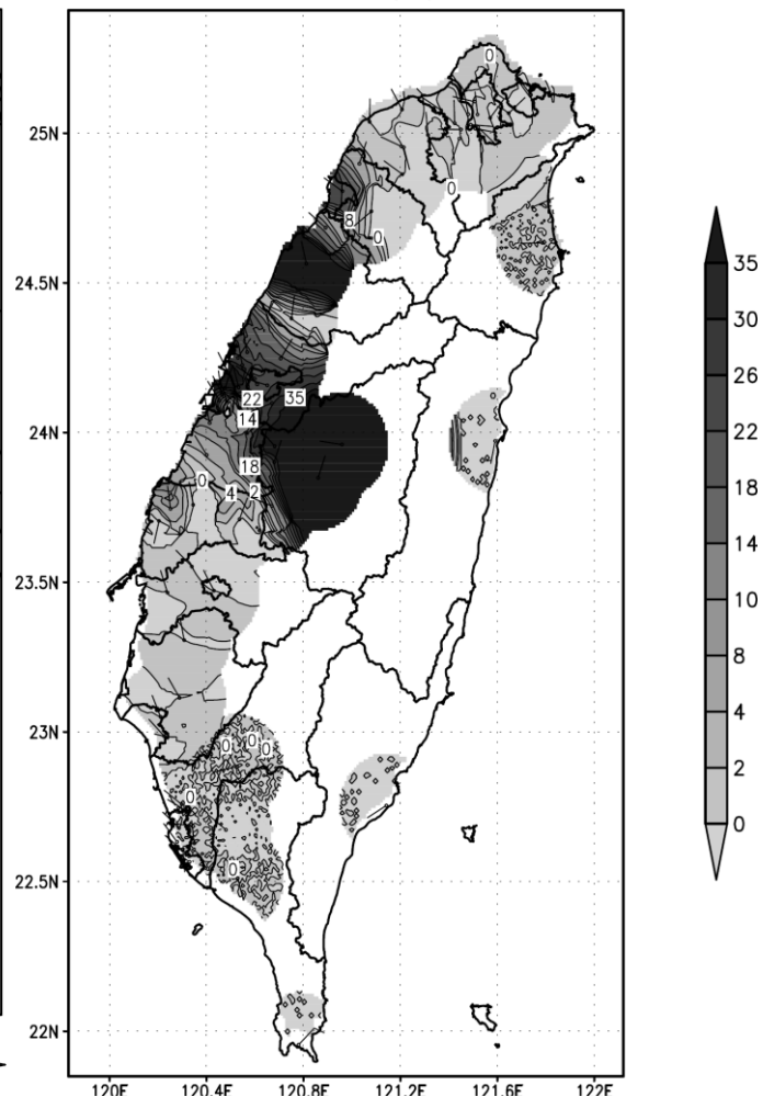
2015 年 11 月 08 日台中電廠+通霄電廠細懸浮微粒貢獻比例圖(事件日)
