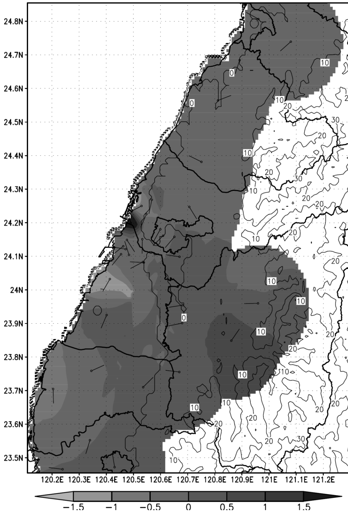
2015-(2010~2014)年 11 月平均風速差值圖(單位：m/s)
