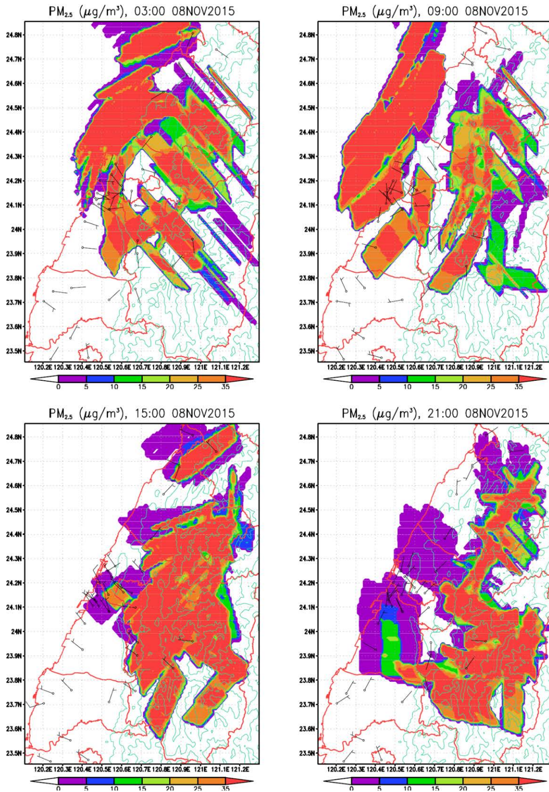
2015 年 11 月 08 日台中火力電廠、通霄火力電廠 3、9、15、21 時 之中部地區距地 20m 細懸浮粒濃度煙線圖 (事件日)
