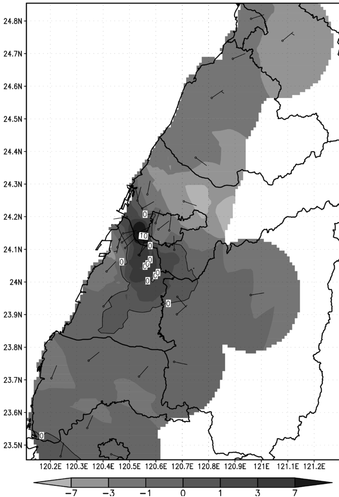
2013-(2008~2012)年9月NO x 月均值之濃度差值圖(單位：ppb)
