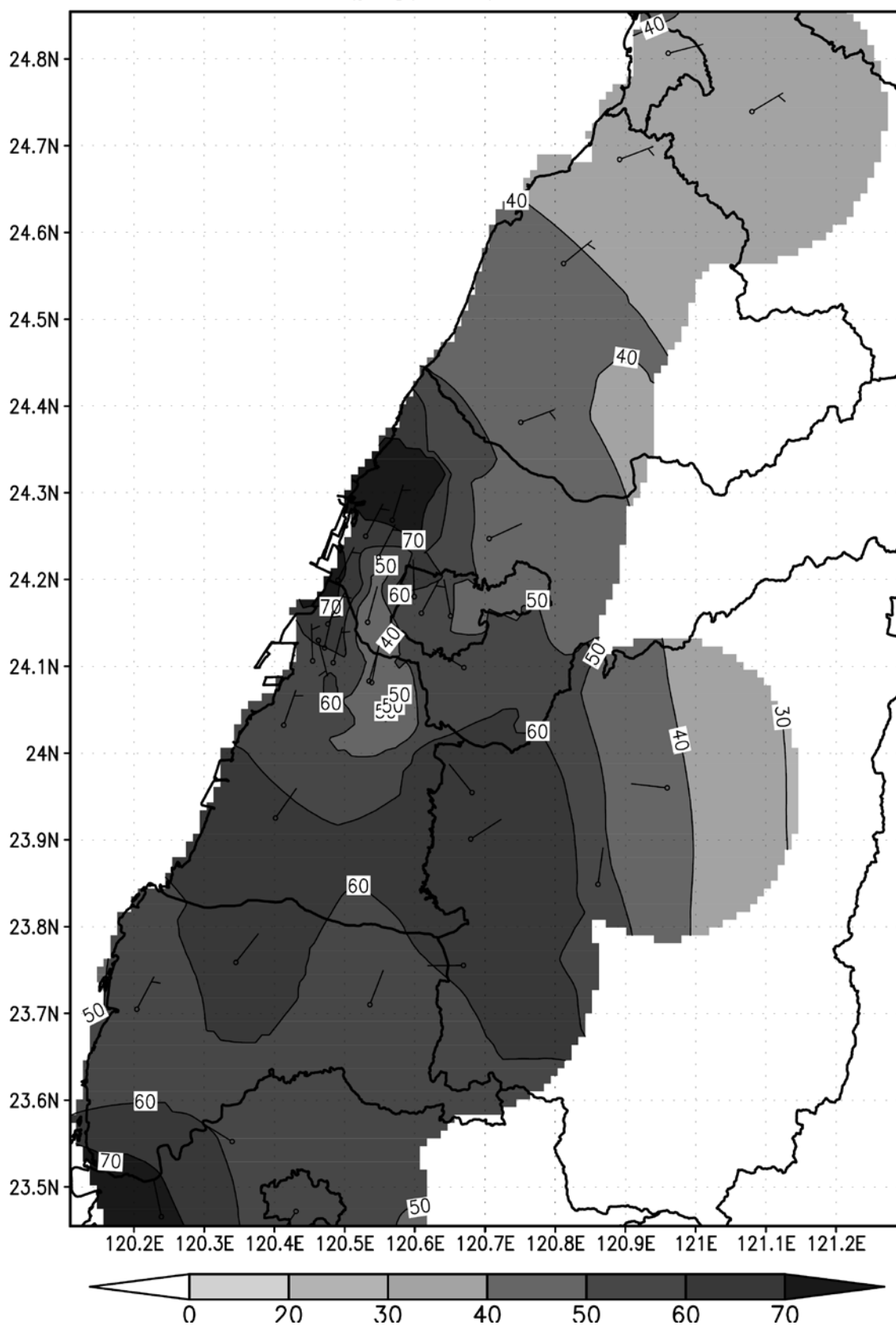
2013 年 9 月份風場及PM 10 ( \mu\text{g}/\text{m}^3 ) 月均值等濃度圖
