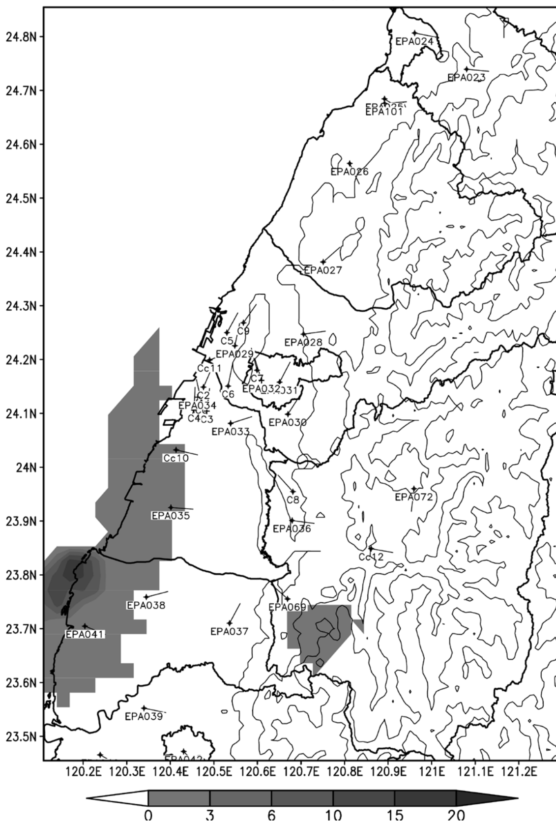
2013 年 9 月 22 日六輕工業區細懸浮微粒貢獻比例圖(非事件日)
