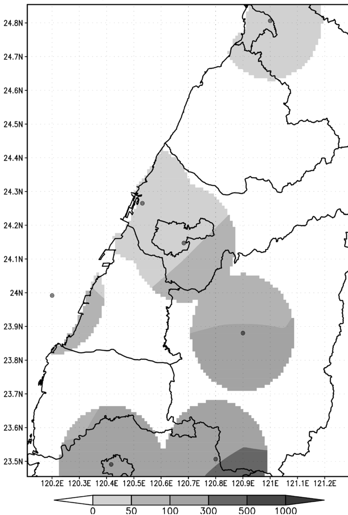
2013 年 9 月份風場及累積雨量(mm)圖
