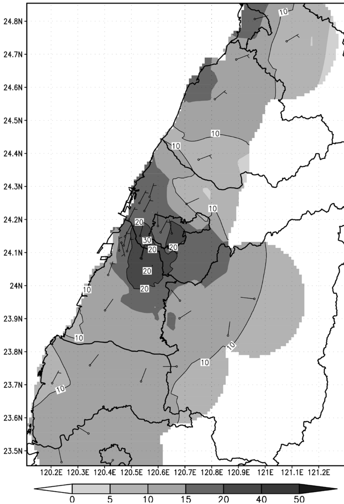
2013 年 9 月份風場及NO x (ppb) 月均值等濃度圖
