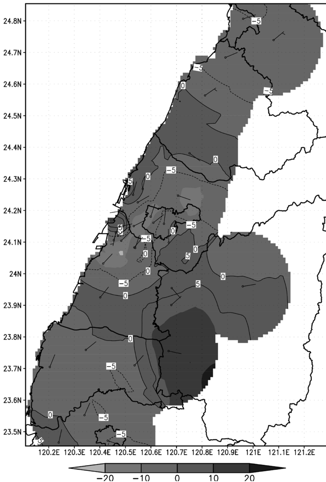
2013-(2008~2012)年 9 月 PM 10 月均值之濃度差值圖(單位： \mu\text{g}/\text{m}^3 )
