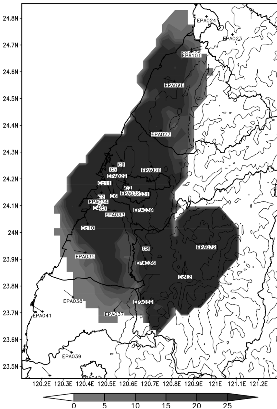
2013 年 9 月 11 日台中火力電廠細懸浮微粒貢獻比例圖(事件日)
