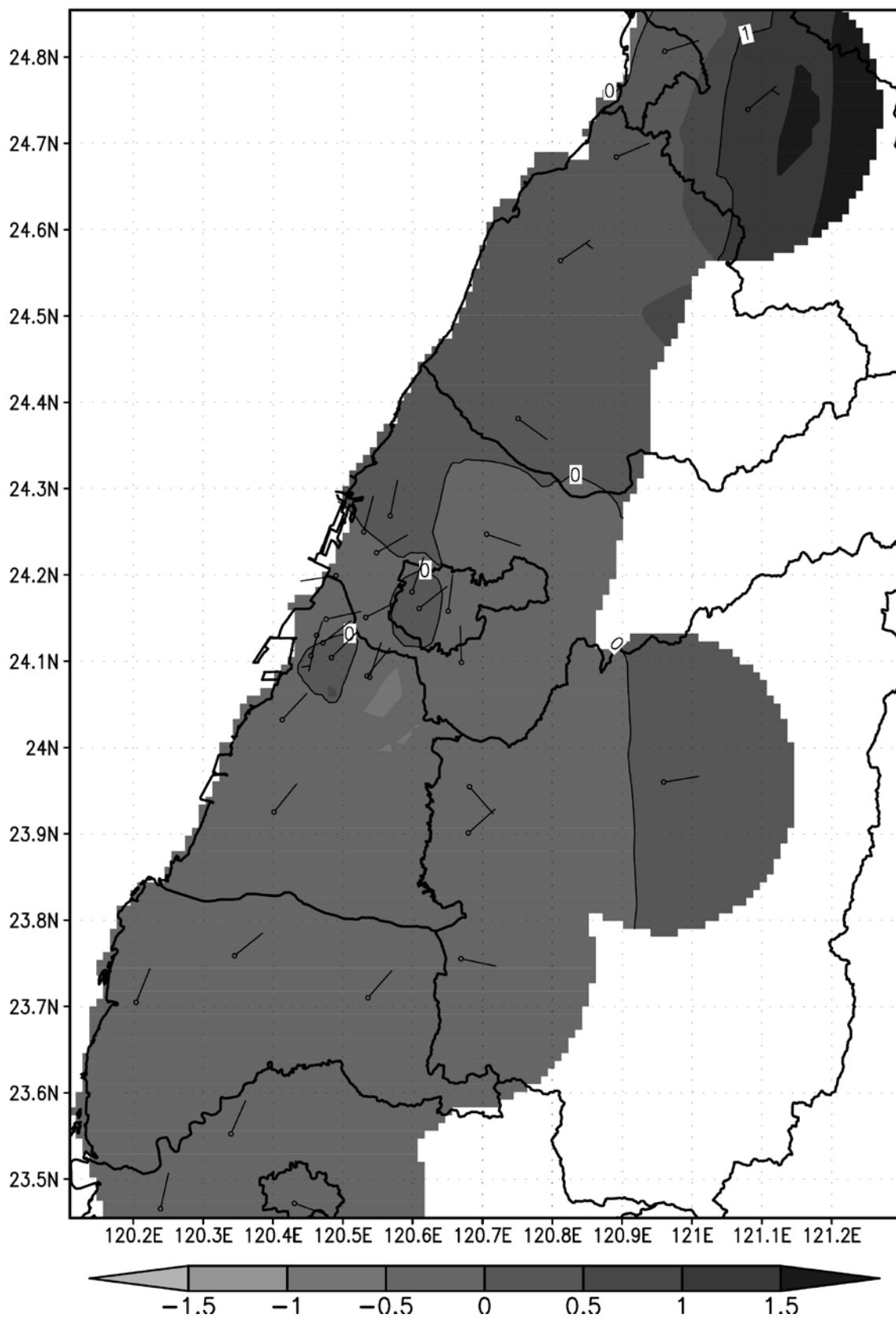
2013-(2008~2012)年9月平均風速差值圖(單位：m/s)
