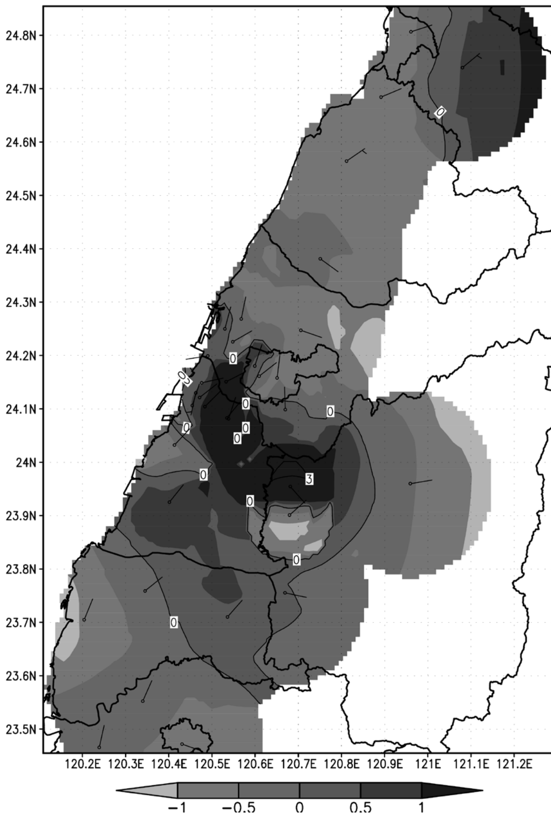
2013-(2008~2012)年 9 月 SO 2 月均值之濃度差值圖(單位：ppb)
