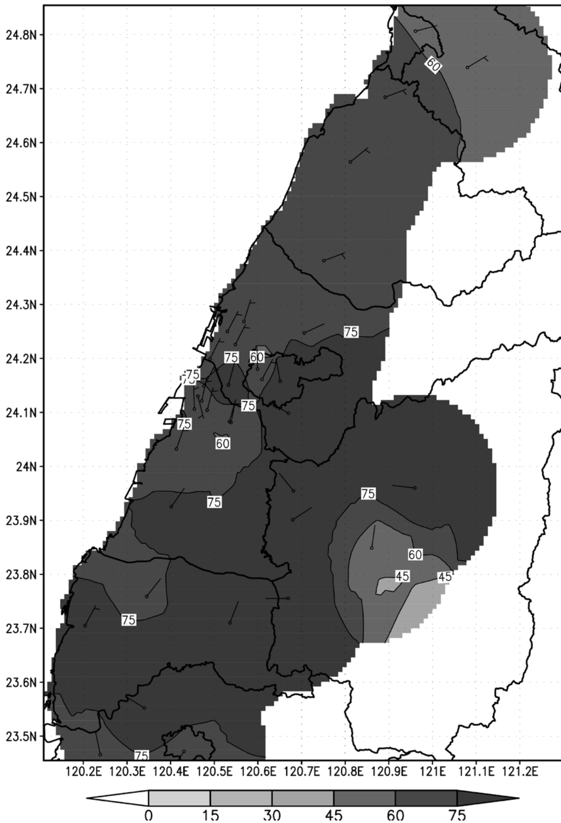
2013 年 9 月份風場及O 3 (ppb) 小時最大值等濃度圖
