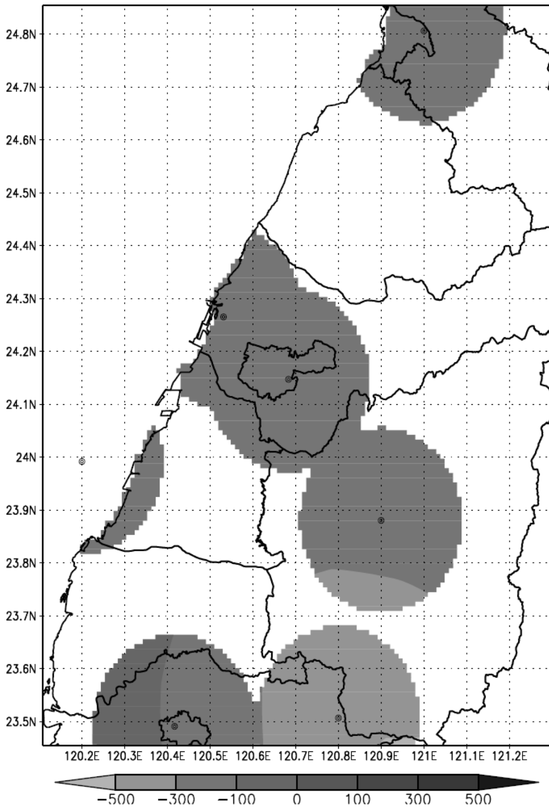
2013-(2008~2012)年9月累積雨量差值圖(單位：mm)
