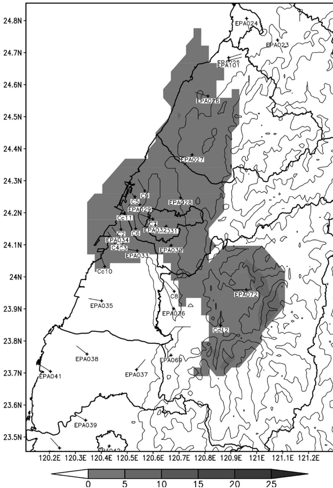
2013 年 9 月 11 日通霄火力電廠細懸浮微粒貢獻比例圖(事件日)
