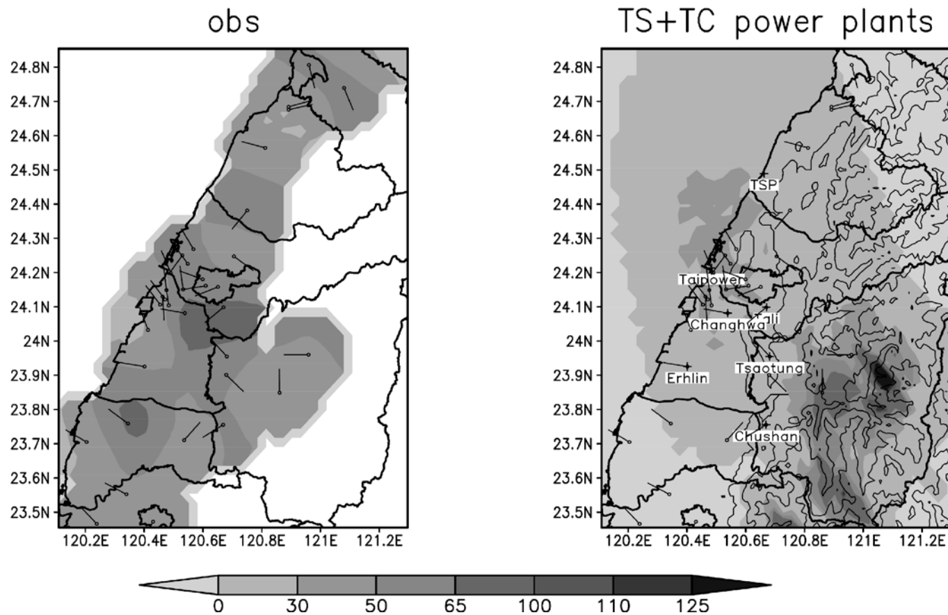
2013 年 9 月 11 日中部地區細懸浮微粒日均值濃度圖及濃度煙線日均值圖(事件日)
