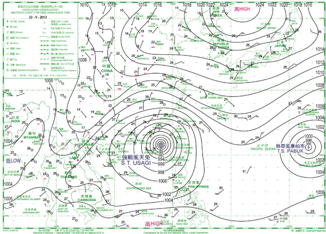
2013 年 9 月 22 日地面天氣圖(非事件日)
