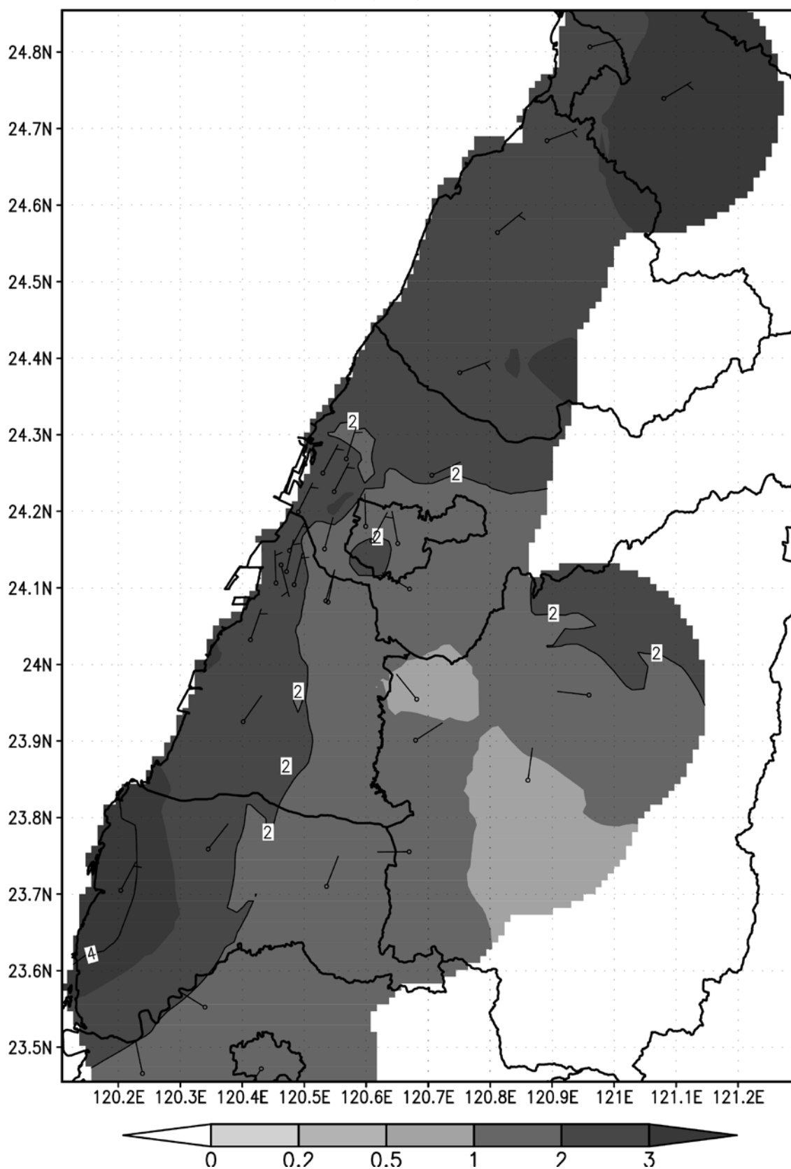
2013 年 9 月份風場及平均風速(m/s)等值圖
