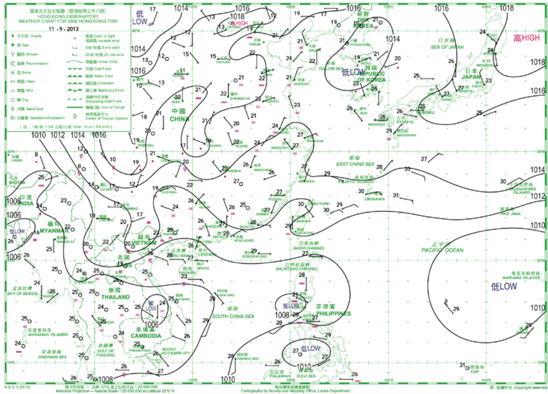
2013 年 9 月 11 日地面天氣圖(事件日)
