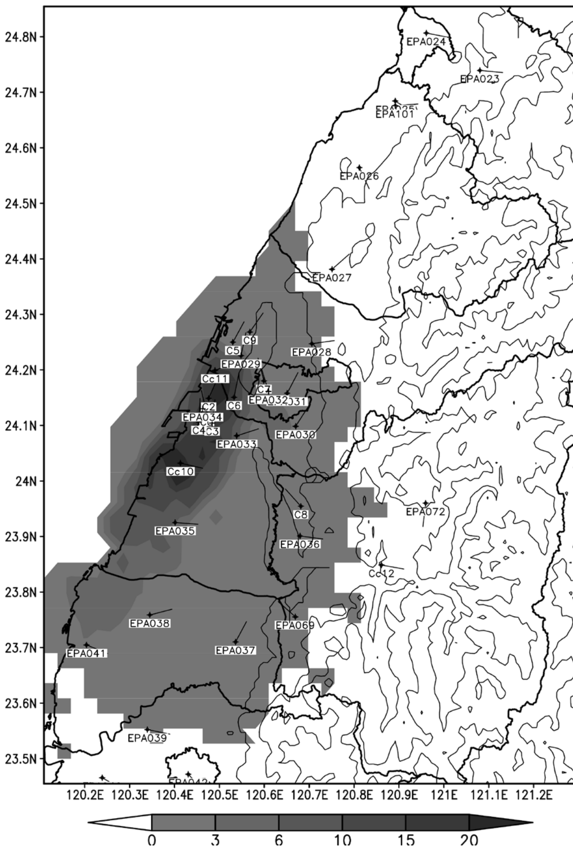
2013 年 9 月 22 日台中火力電廠細懸浮微粒貢獻比例圖(非事件日)
