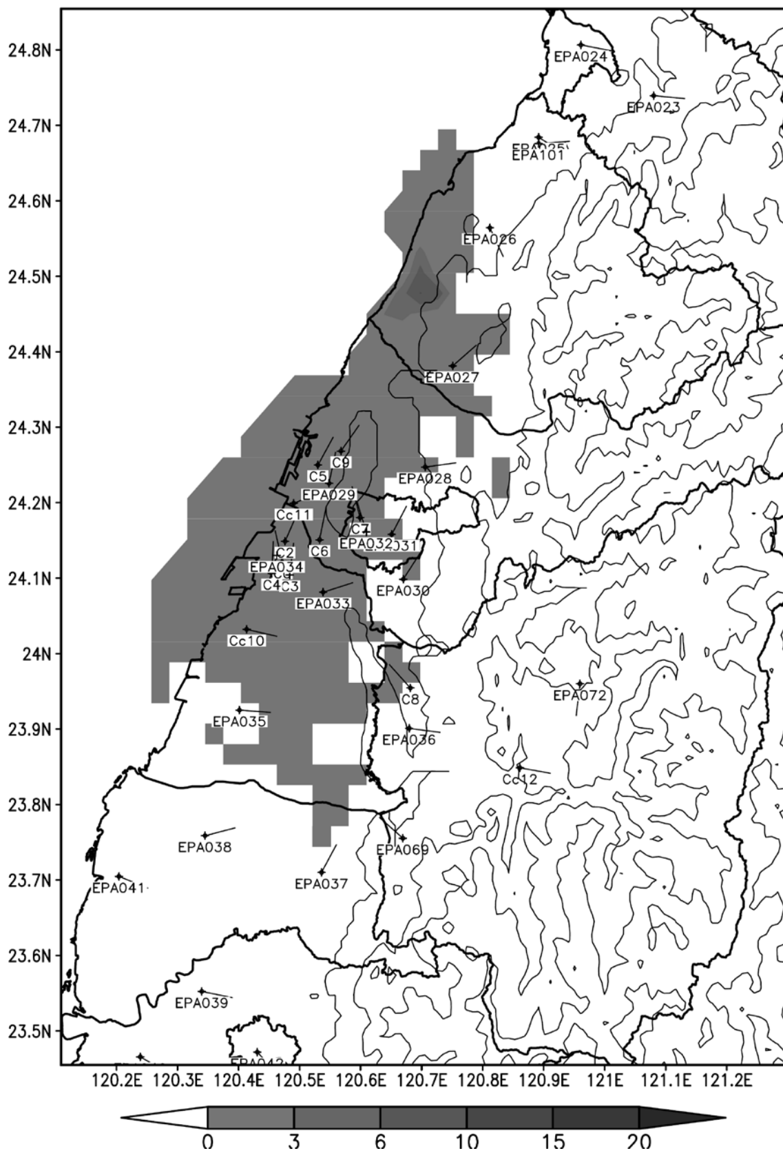
2013 年 9 月 22 日通霄火力電廠細懸浮微粒貢獻比例圖(非事件日)
