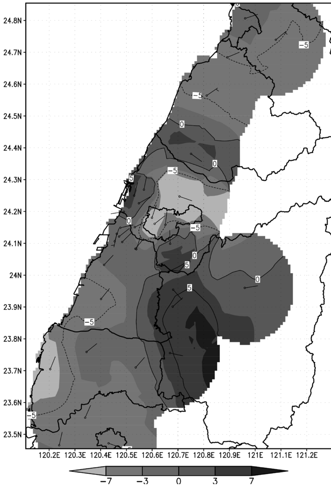
2013-(2008~2012)年 9 月 PM_{2.5} 月均值之濃度差值圖(單位： \mu g/m^3 )
