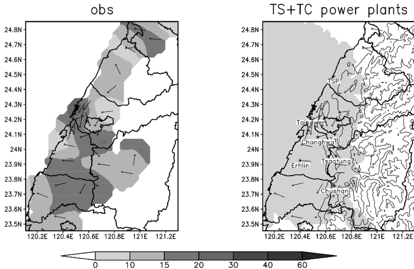
2013 年 9 月 22 日中部地區細懸浮微粒日均值濃度圖及濃度煙線日均值圖(非事件日)
