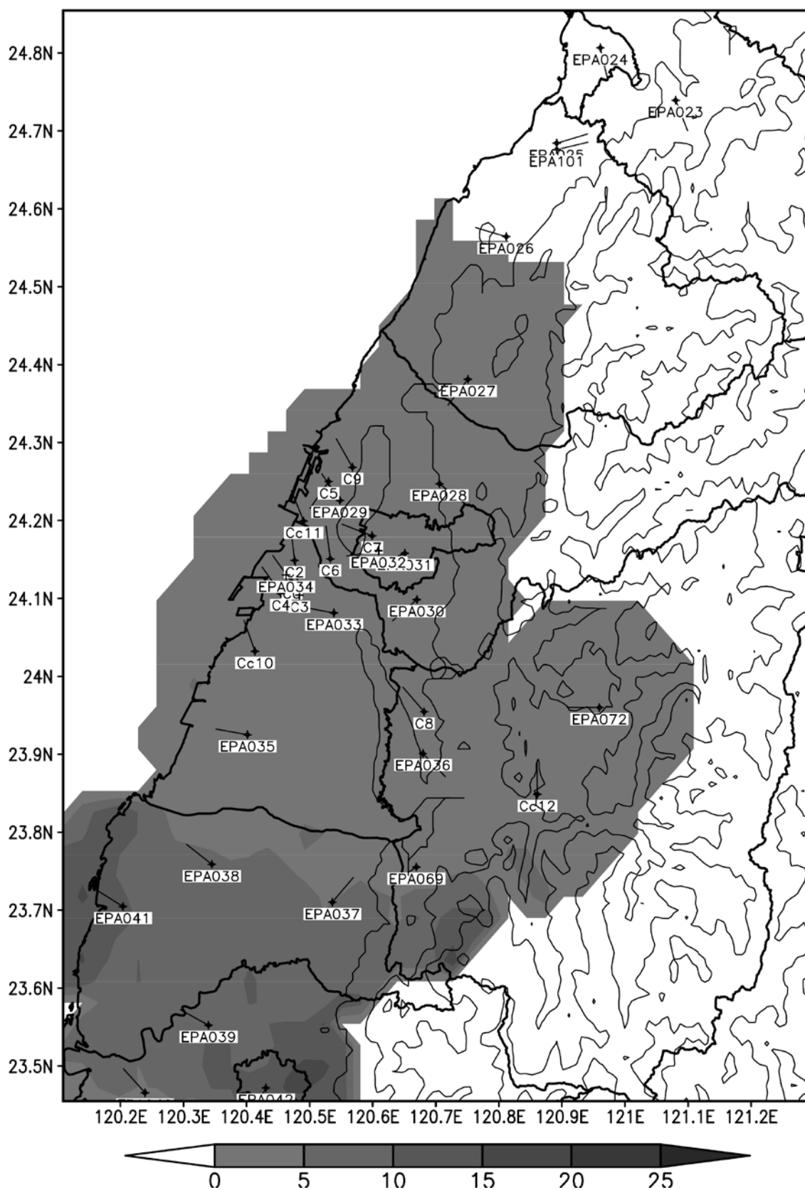
2013 年 9 月 11 日六輕工業區細懸浮微粒貢獻比例圖(事件日)
