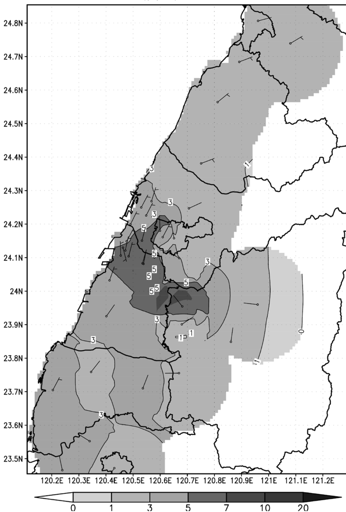
2013 年 9 月份風場及SO 2 (ppb) 月均值等濃度圖
