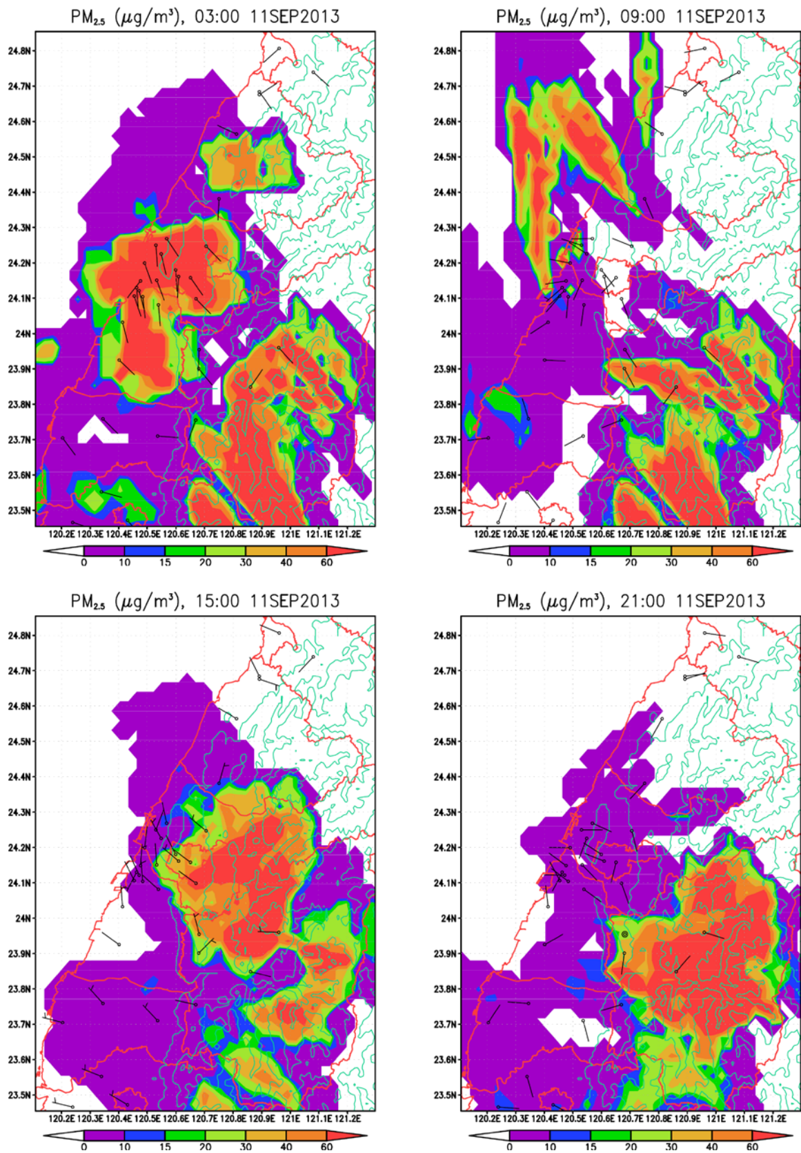
2013 年 9 月 11 日 台中火力電廠、通霄火力電廠及六輕工業區 3、9、15、21 時 之距地 20m 細懸浮粒濃度煙線圖 (事件日)
