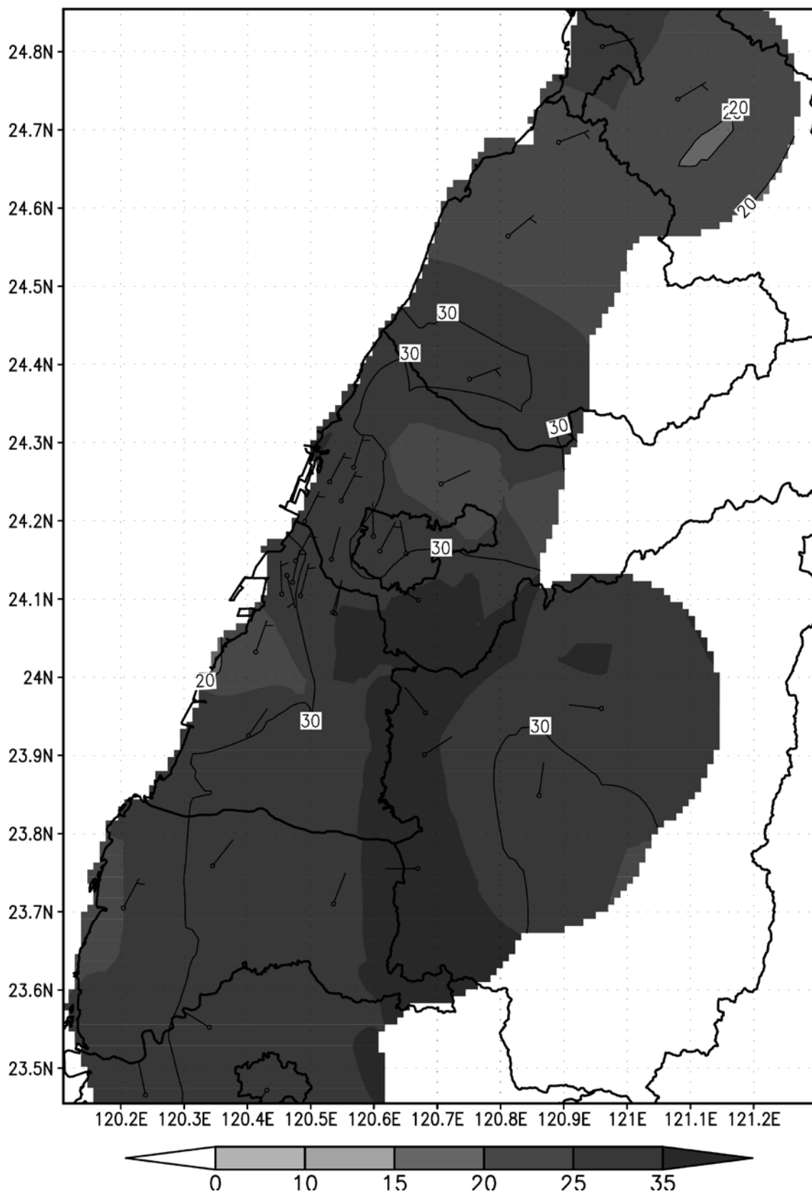
2013 年 9 月份風場及PM 2.5 ( \mu\text{g}/\text{m}^3 ) 月均值等濃度圖
