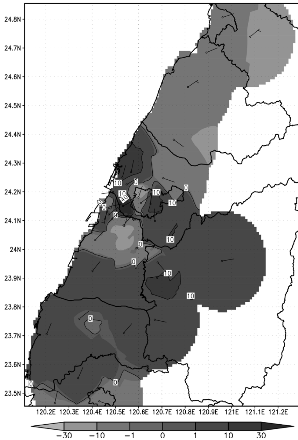
2013-(2008~2012)年9月O 3 小時最大值之濃度差值圖(單位：ppb)
